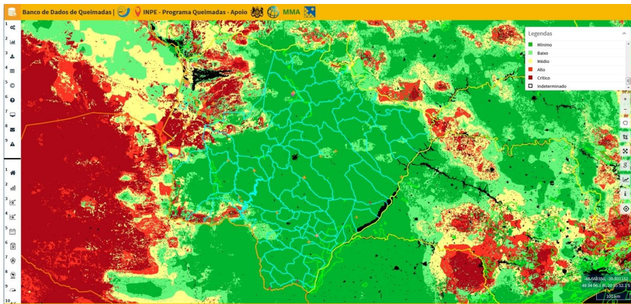
Mapa 1. Risco de fogo no Estado de Mato Grosso do Sul. FONTE: INPE, 15/04/2020.
