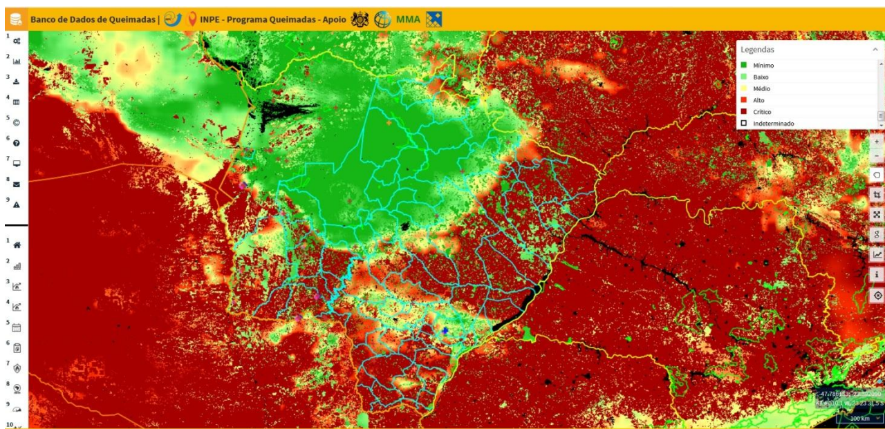
Mapa 1. Risco de fogo observado em 20/05/2020 no Estado de Mato Grosso do Sul. FONTE: INPE.
