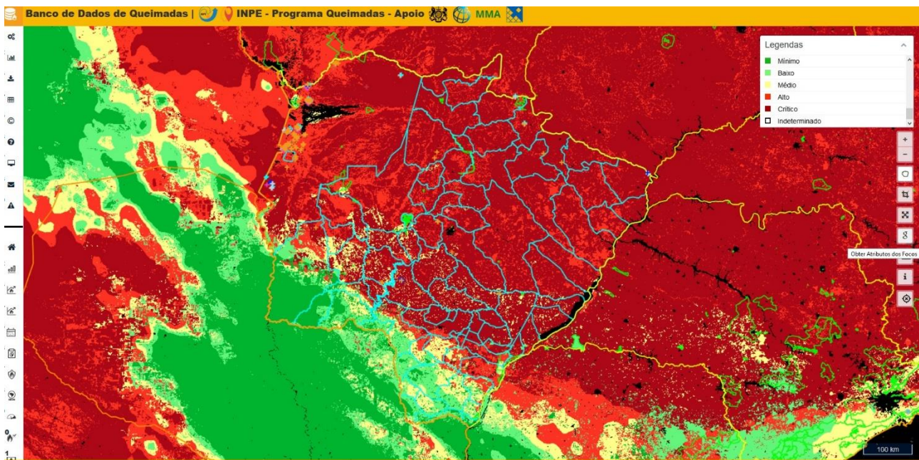
Mapa 1. Risco de fogo observado em 27/07/2020 no Estado de Mato Grosso do Sul. FONTE: INPE.
