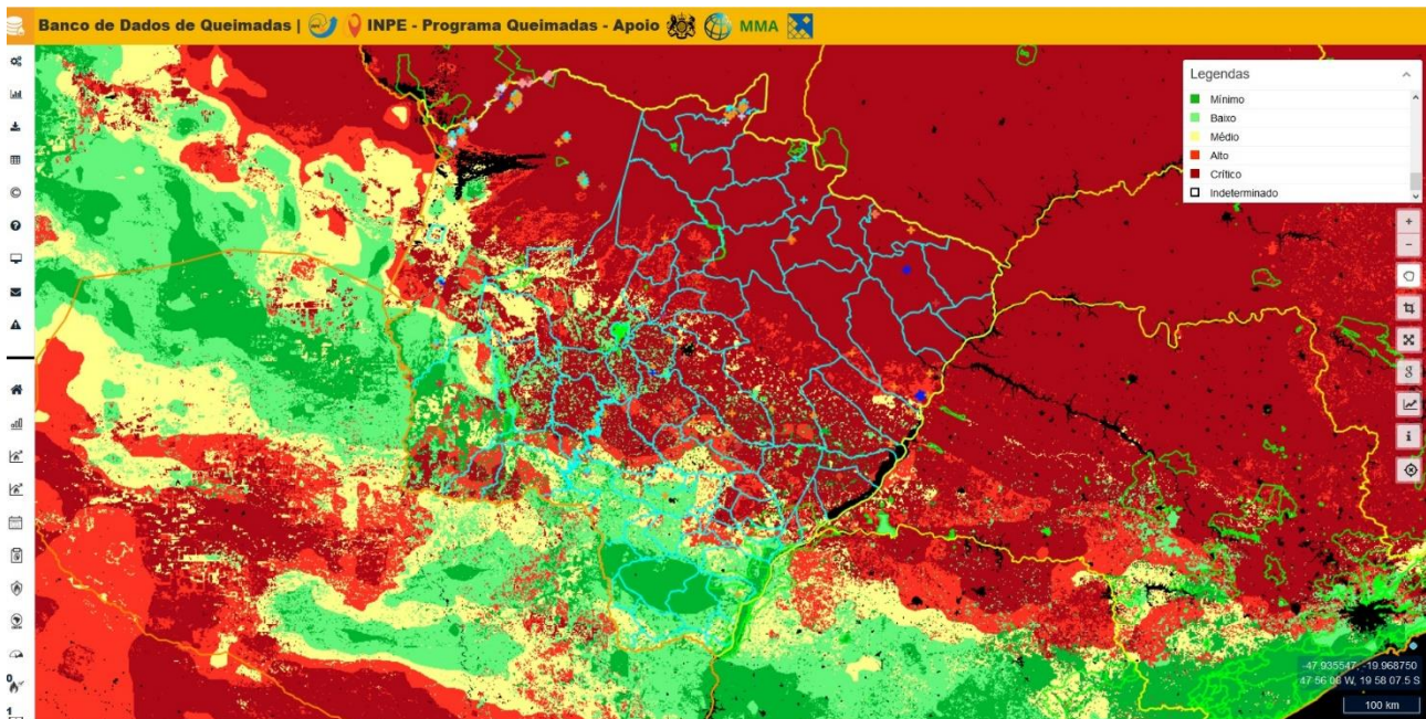
Mapa 1. Risco de fogo observado em 02/09/2020 no Estado de Mato Grosso do Sul. FONTE: INPE.
