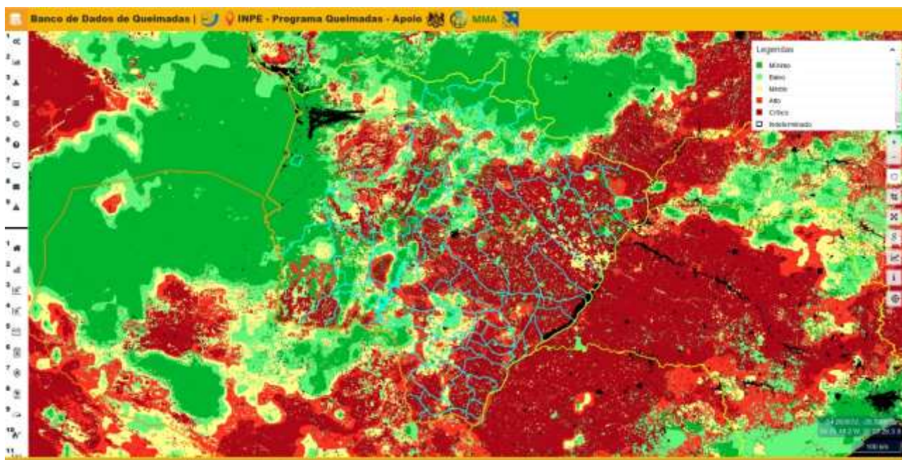
Mapa 1. Risco de fogo observado em 25/10/2020 no Estado de Mato Grosso do Sul. FONTE: INPE.
