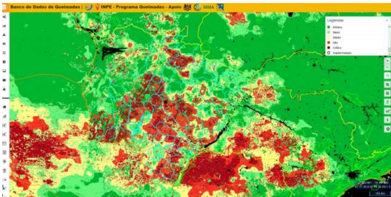
Mapa 1. Risco de fogo observado em 15/12/2020 no Estado de Mato Grosso do Sul. FONTE: INPE.
