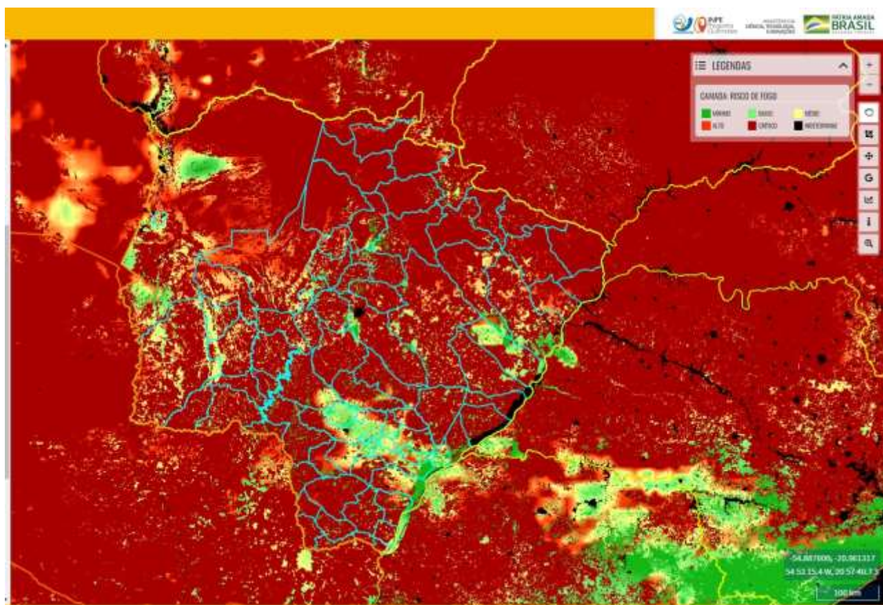
Mapa 1. Risco de fogo observado em 20/09/2021 no Estado de Mato Grosso do Sul. FONTE: INPE.
