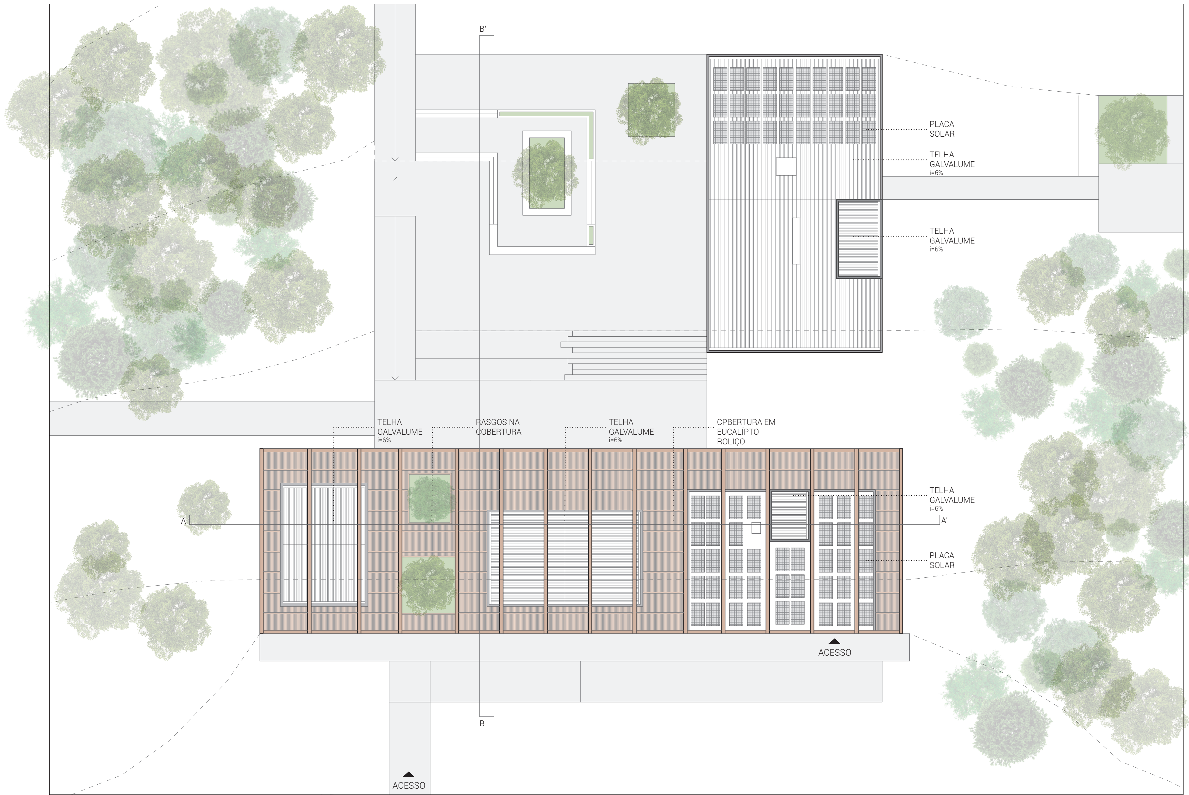
PLANTA COBERTURA DO CENTRO DE VISITANTES DA GRUTA DE LAGO AZUL
