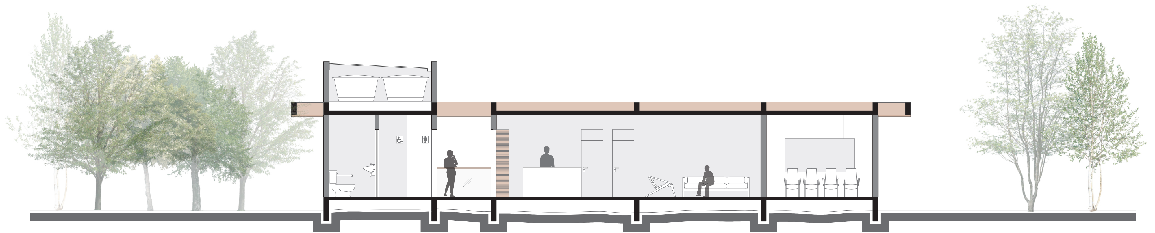
CORTE LONGITUDINAL DO CENTRO DE APOIO AO VISITANTE DA GRUTA DE N. SRA. APARECIDA
