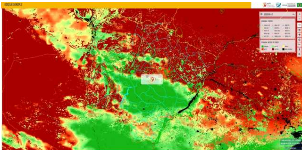
Mapa 1. Risco de fogo observado em 31/08/2022 no Estado de Mato Grosso do Sul. FONTE: INPE.
