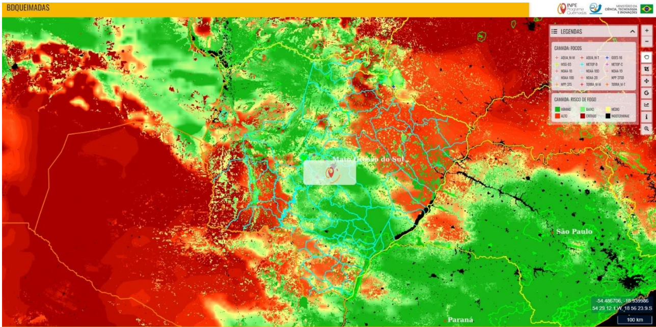
Mapa 1. Risco de fogo observado em 12/08/2022 no Estado de Mato Grosso do Sul. FONTE: INPE.
