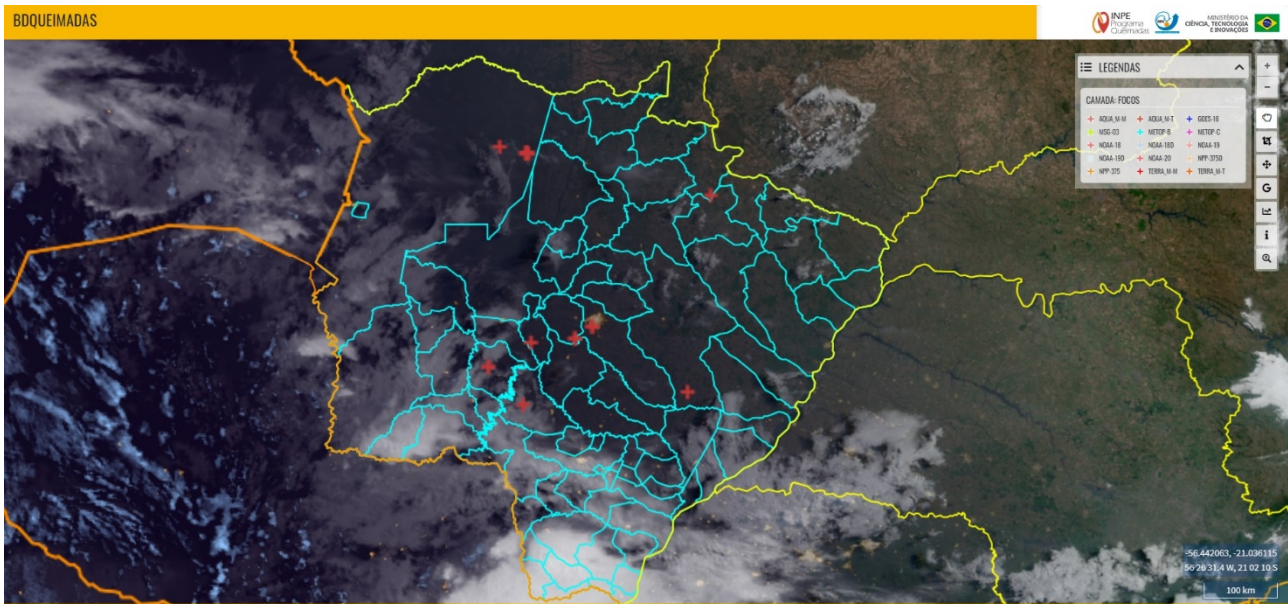
Mapa 1. Risco de fogo observado em 27/07/2023 no Estado de Mato Grosso do Sul. FONTE: INPE.
