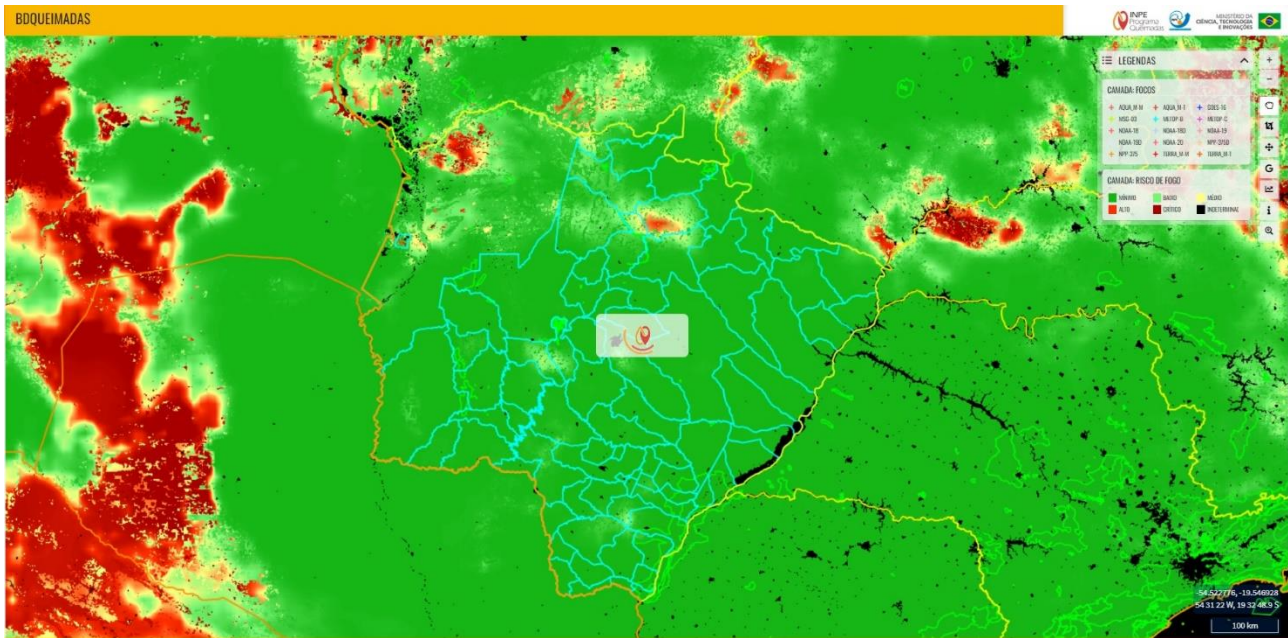
Mapa 1. Risco de Fogo observado em 24/11/2023 no Estado de Mato Grosso do Sul. FONTE: INPE.
