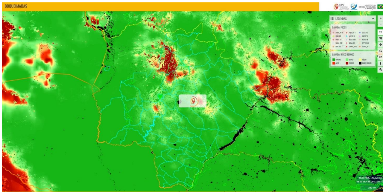
Mapa 1. Risco de Fogo observado em 08/12/2023 no Estado de Mato Grosso do Sul. FONTE: INPE.
