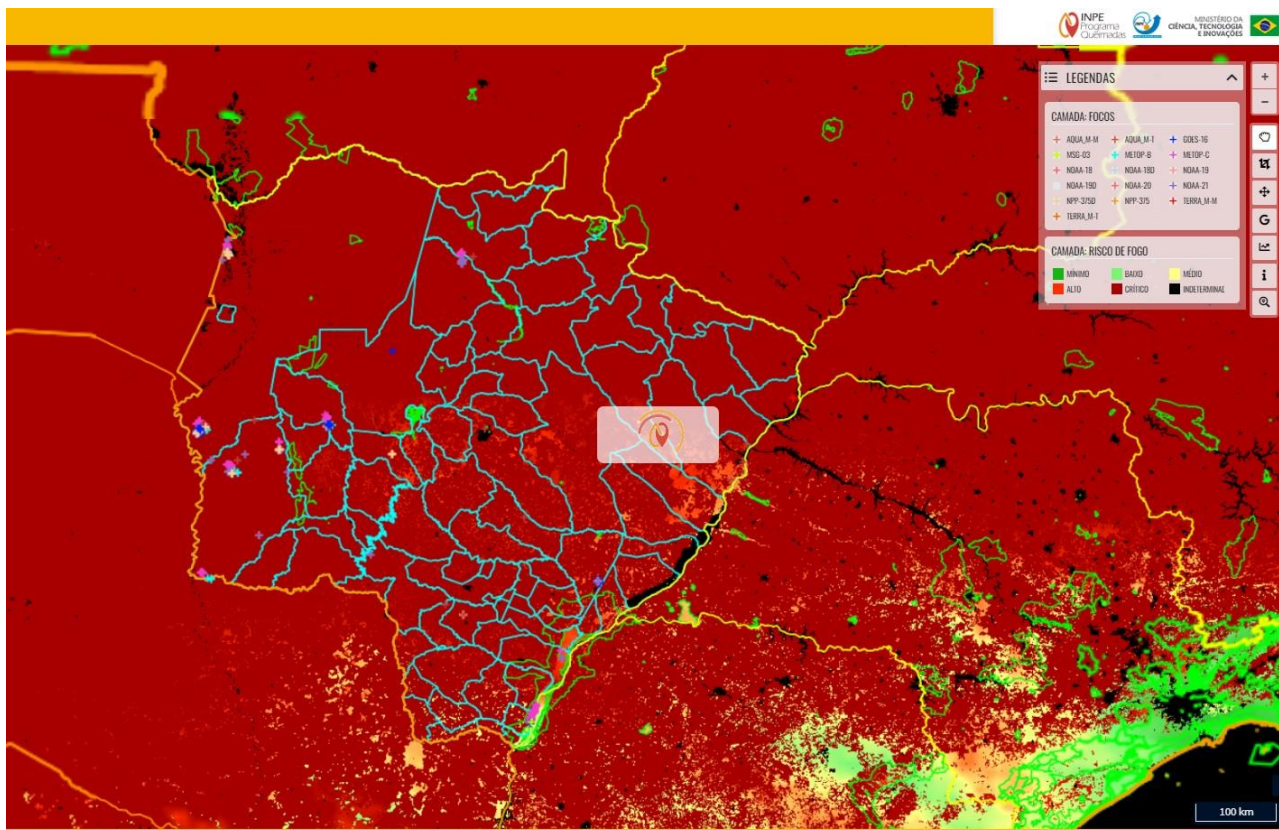
Mapa 1. Risco de Fogo observado em 29/08/2024 no Estado de Mato Grosso do Sul. Fonte: INPE.
