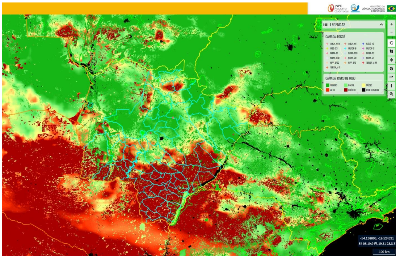
Mapa 1. Risco de Fogo observado em 12/11/2024 no Estado de Mato Grosso do Sul. Fonte: INPE.
