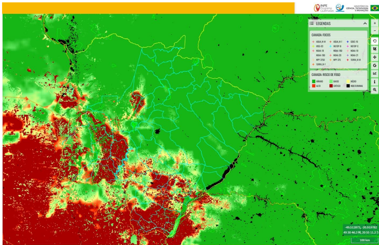
Figura 1. Risco de Fogo observado em 04/02/2025 no Estado de Mato Grosso do Sul. Fonte: INPE.
