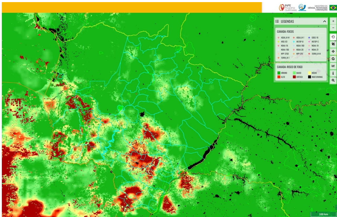
Figura 1. Risco de Fogo observado em 10/02/2025 no Estado de Mato Grosso do Sul. Fonte: INPE.
