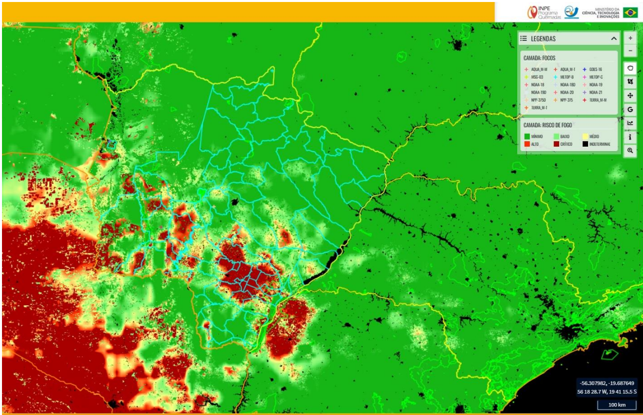
Figura 1. Risco de Fogo observado em 13/02/2025 no Estado de Mato Grosso do Sul. Fonte: INPE.
