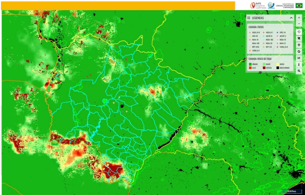
Figura 1. Risco de Fogo observado em 19/02/2025 no Estado de Mato Grosso do Sul. Fonte: INPE.
