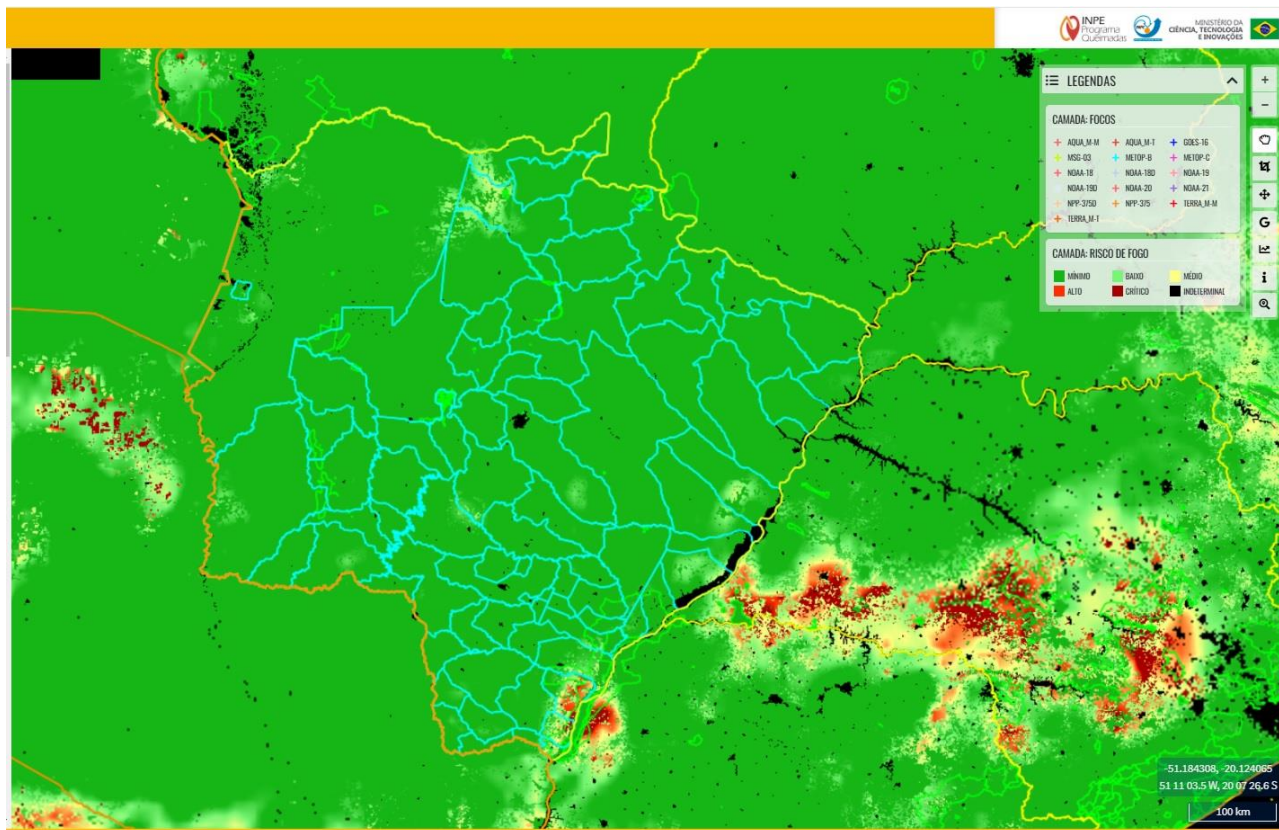
Figura 1. Risco de Fogo observado em 27/02/2025 no Estado de Mato Grosso do Sul. Fonte: INPE.
