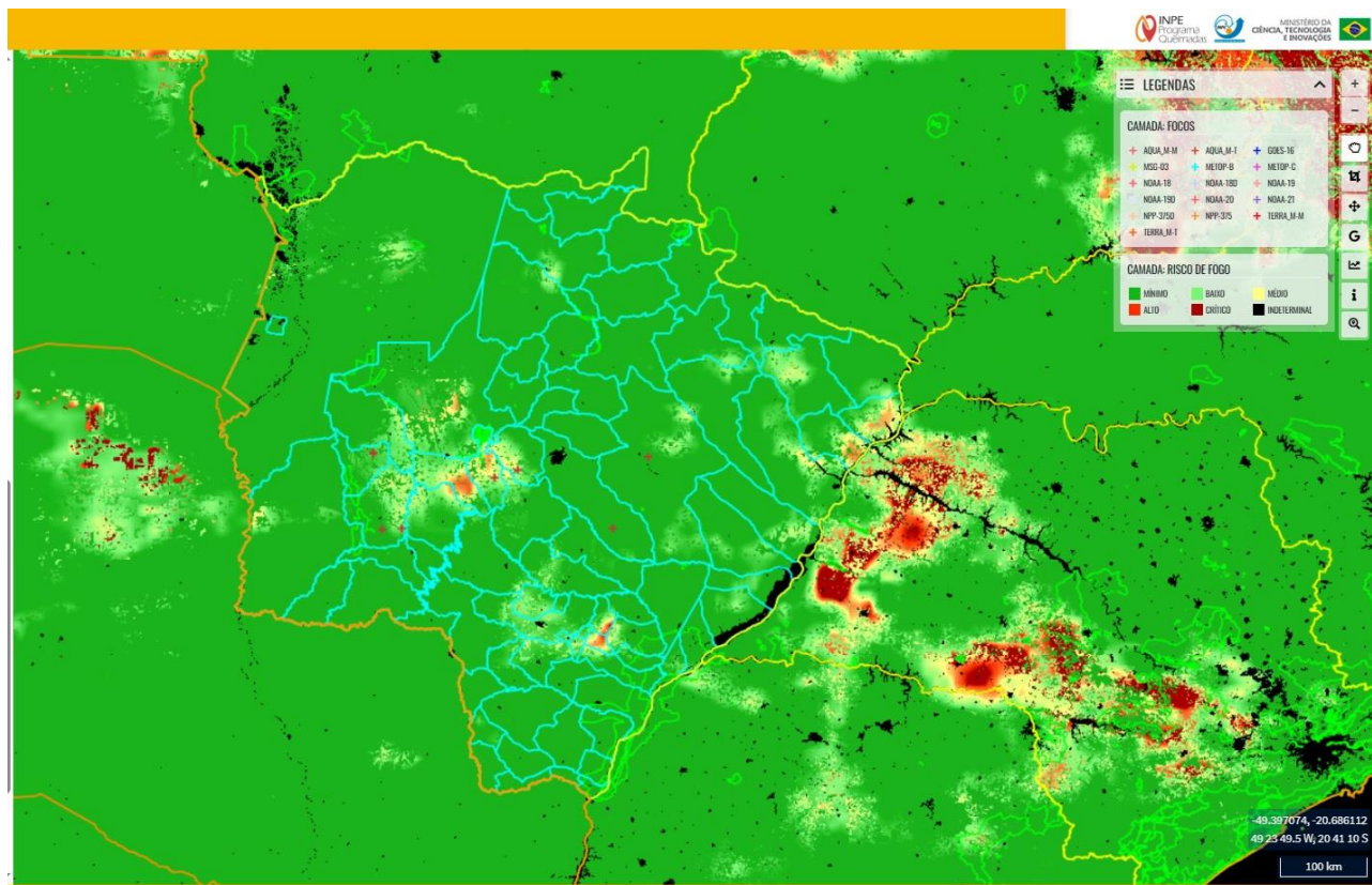
Figura 1. Risco de Fogo observado em 19/03/2025 no Estado de Mato Grosso do Sul. Fonte: INPE.
