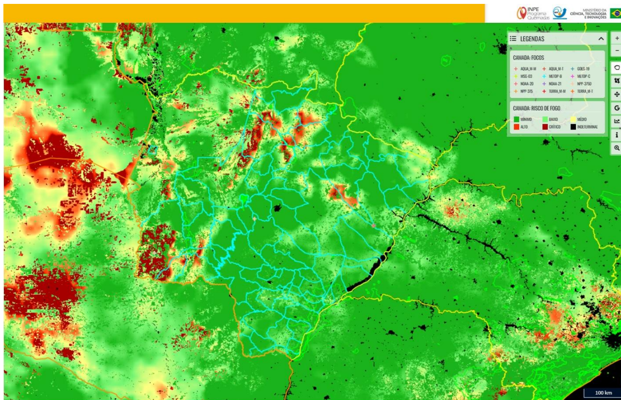
Figura 1. Risco de Fogo observado em 08/01/2026 no Estado de Mato Grosso do Sul. Fonte: INPE.
