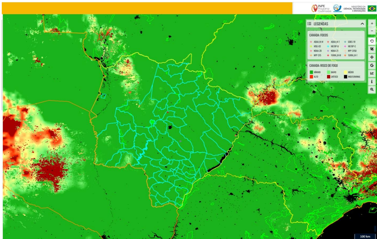
Figura 1. Risco de Fogo observado em 13/01/2026 no Estado de Mato Grosso do Sul. Fonte: INPE.
