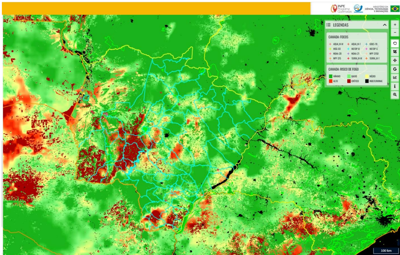
Figura 1. Risco de Fogo observado em 27/01/2026 no Estado de Mato Grosso do Sul. Fonte: INPE.
