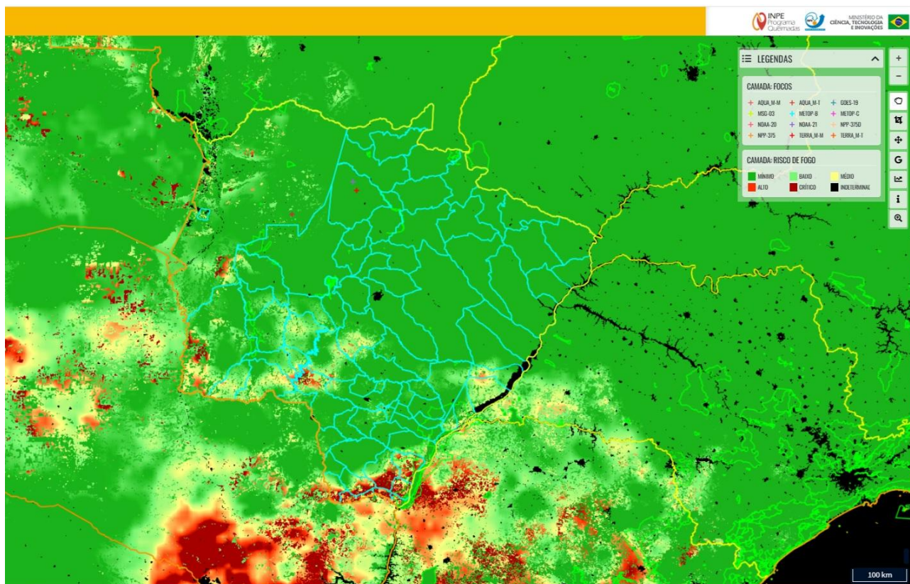
Figura 1. Risco de Fogo observado em 13/02/2026 no Estado de Mato Grosso do Sul. Fonte: INPE.
