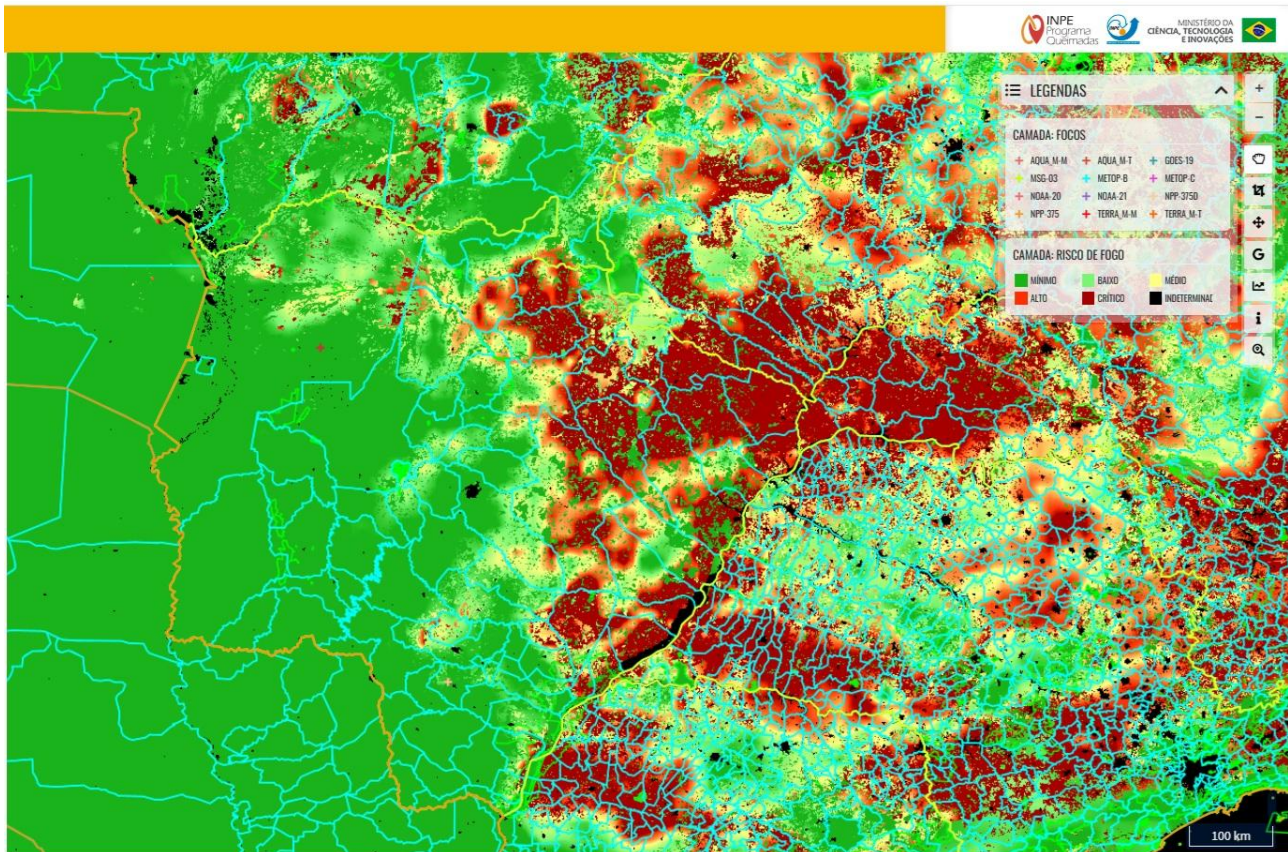
Figura 1. Risco de Fogo observado em 22/04/2026 no Estado de Mato Grosso do Sul. Fonte: INPE.
